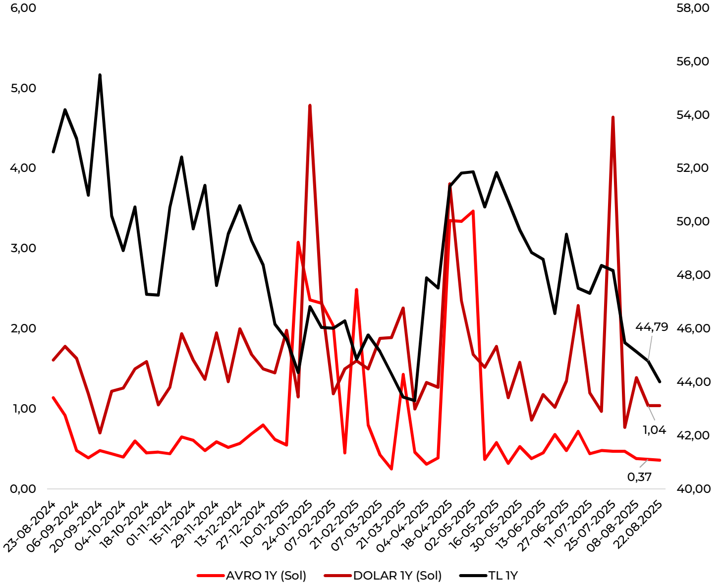
Grafik-5: Mevduat Faizi İstatistikleri (seviye, akım)
