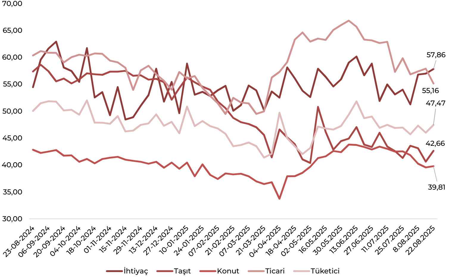
Grafik-4: Kar Payı İstatistikleri (akım, seviye, %)
