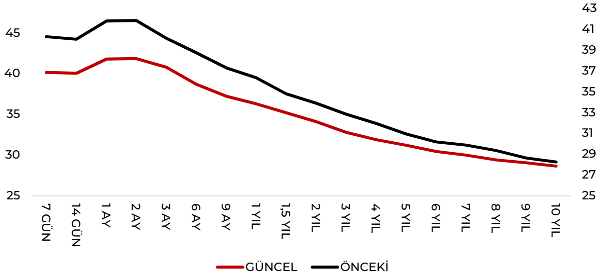
Grafik-1: Swap Eğrisi (seviye, %, 29 Eylül 2025)
